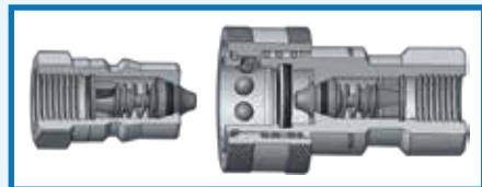
(A+B) ISO hydrauliek koppeling
