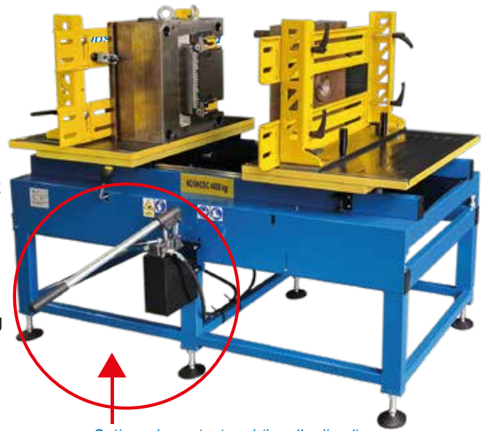
Optioneel gepatenteerd (handbediend) hydraulisch opening systeem
